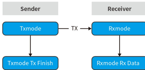
图 7.1 Basic 模式通信示意图
