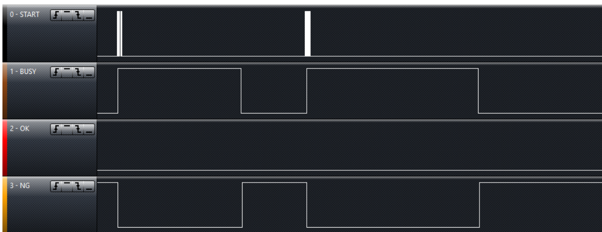
失败实际逻辑分析仪截图：
